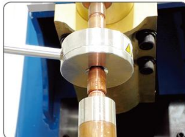
负荷传感器下部照片
